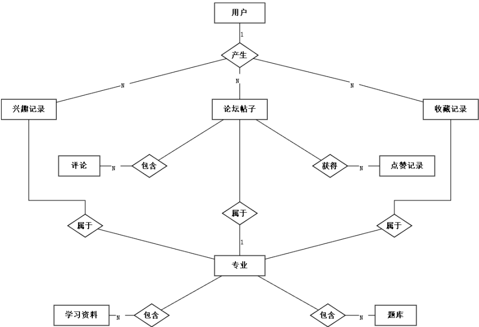
图 4-5 用户相关 E-R 图
