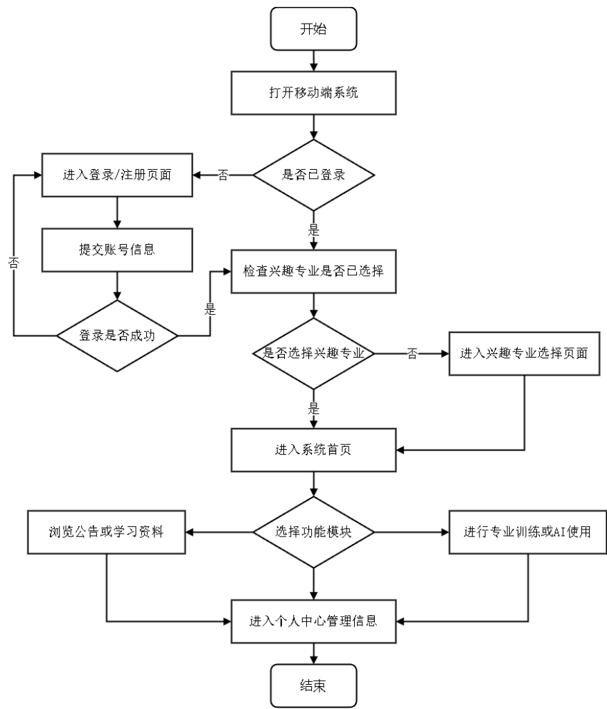
图 3-4 用户使用流程图
