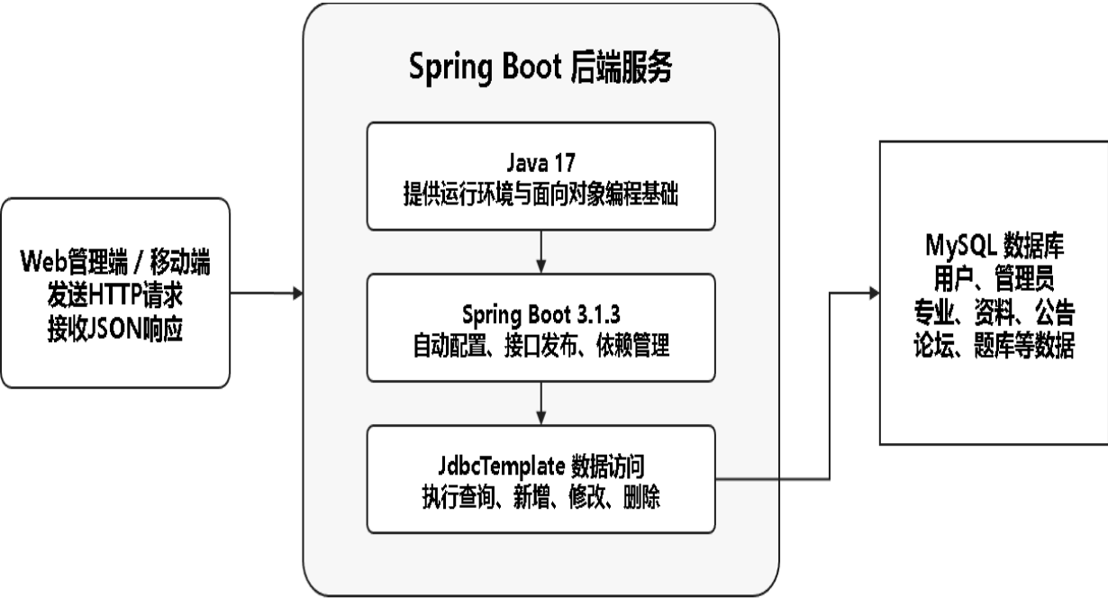
图 2-1 后端开发技术关系图
