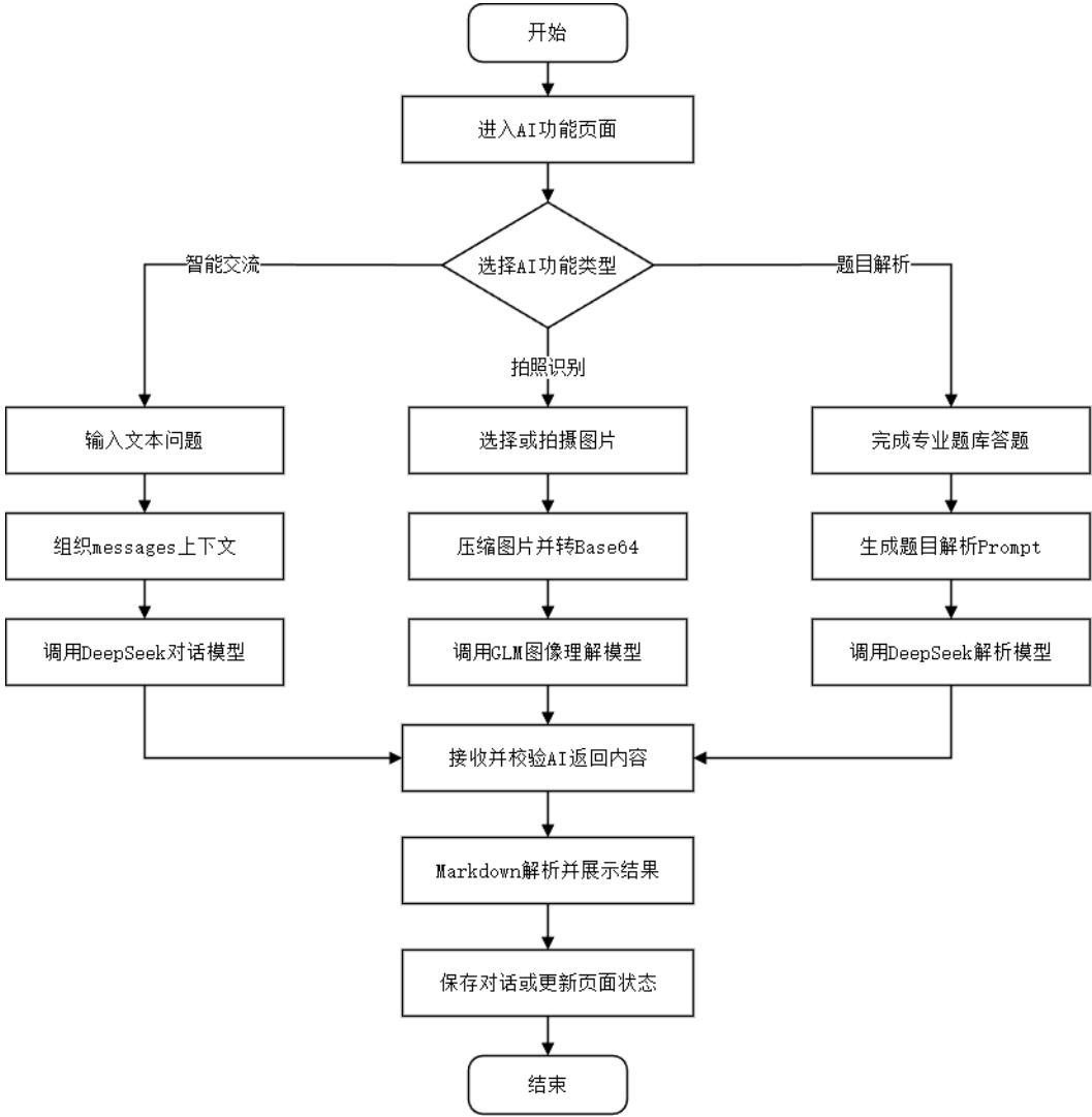
图 5-10 AI 功能模块详细流程图
