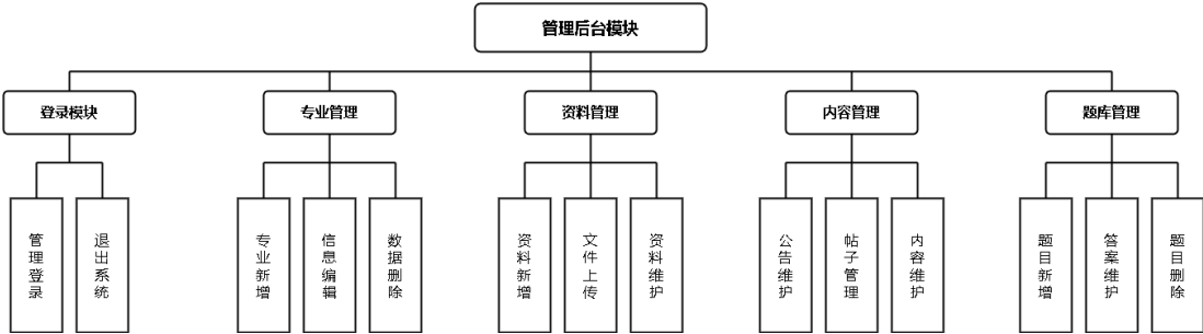
图 4-2 管理后台模块功能结构图
