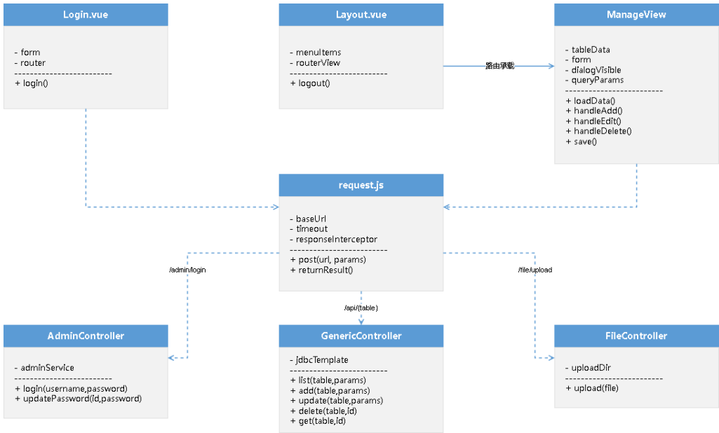
图 5-1 管理后台模块类图
