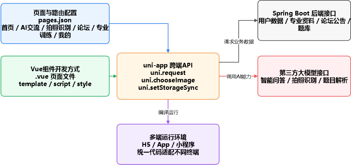
图 2-2 uni-app 框架运行关系图
