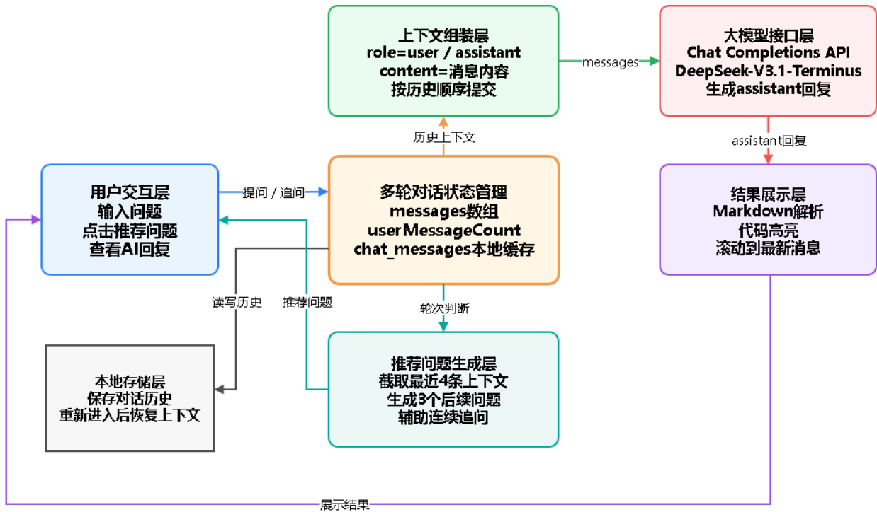
图 2-3 多轮对话技术关系图
