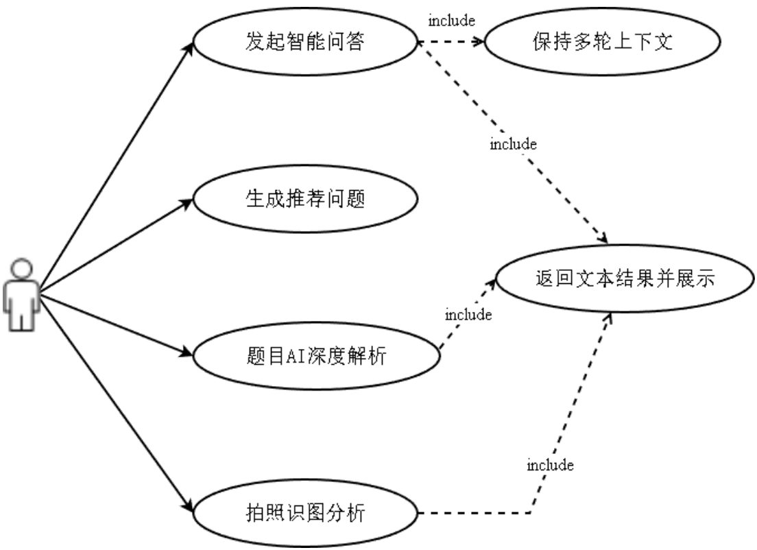
图 3-3 AI 功能用例图
