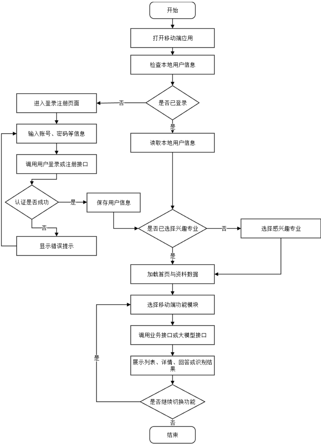
图 5-6 用户移动端详细流程图
