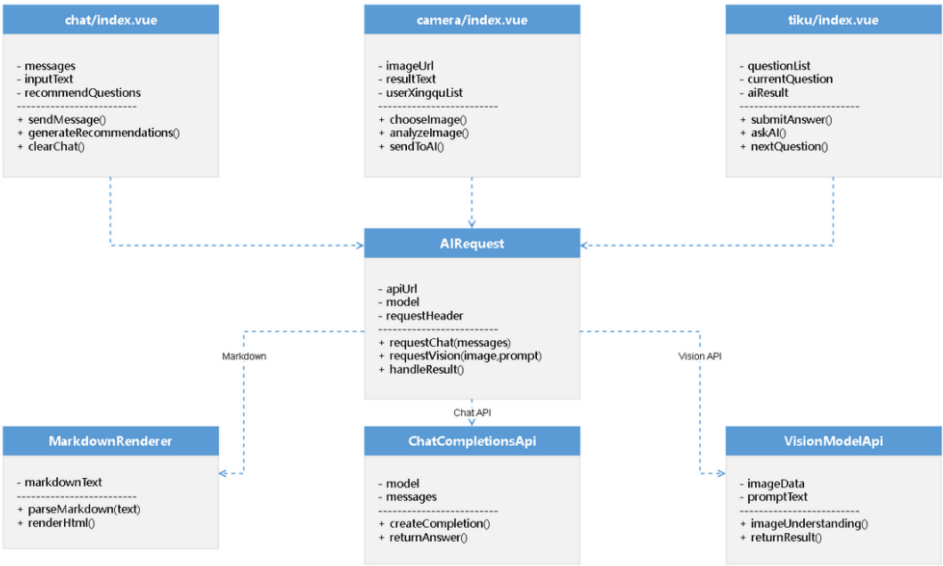
图 5-9 AI 功能模块类图
