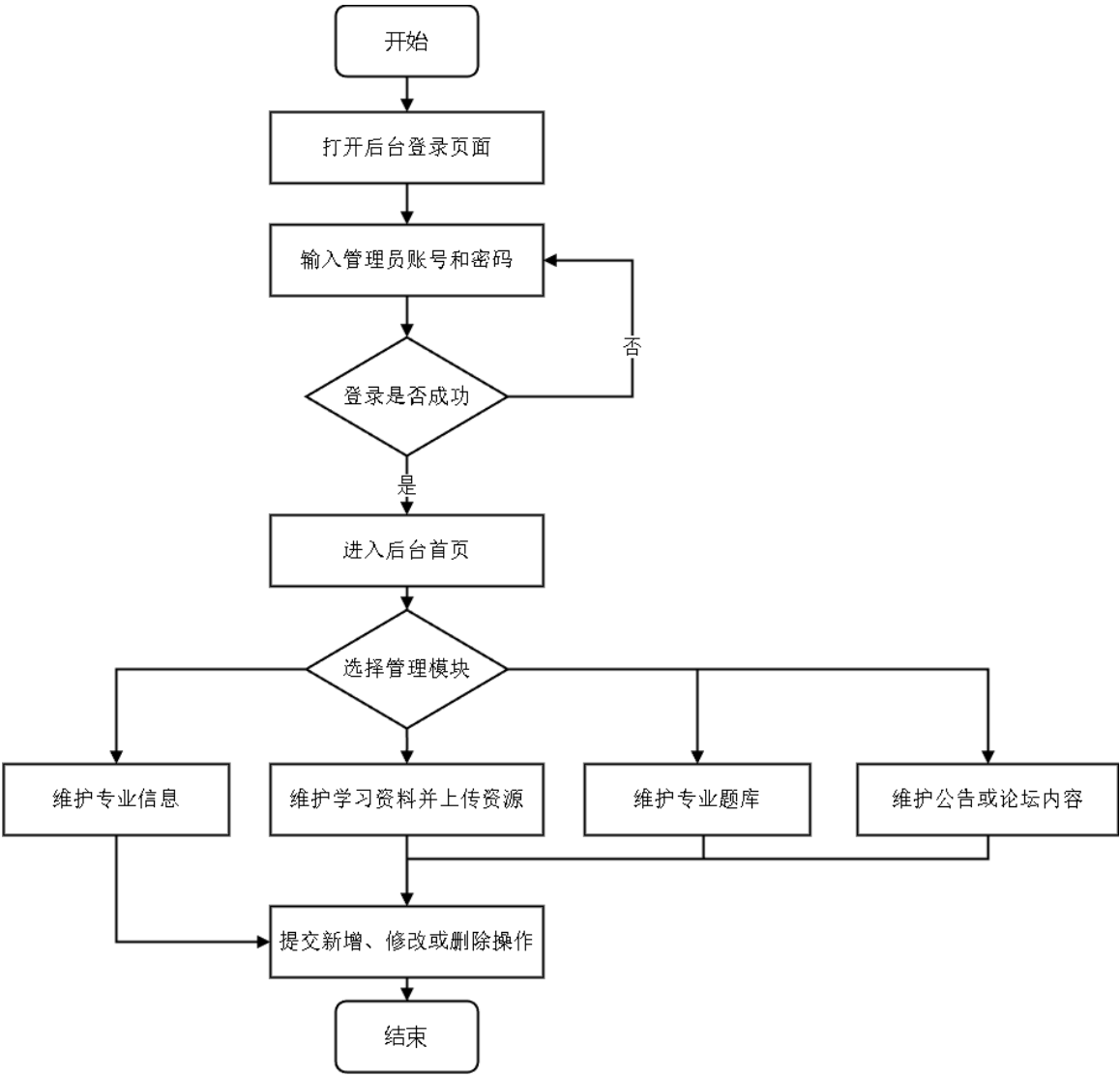
图 3-5 管理员管理流程图
