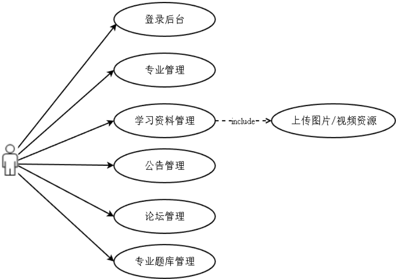
图 3-1 管理员端功能用例图
