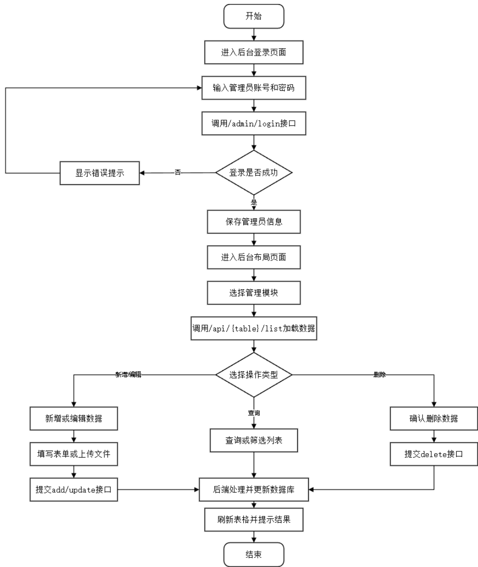
图 5-2 管理后台模块详细流程图
