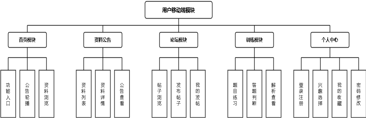
图 4-3 用户移动端模块功能结构图
