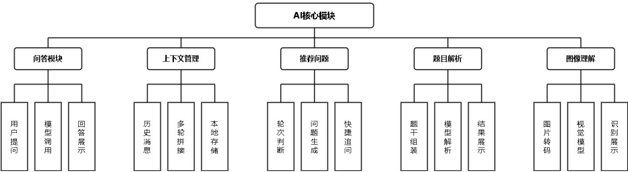
图 4-4 AI 核心模块功能结构图
