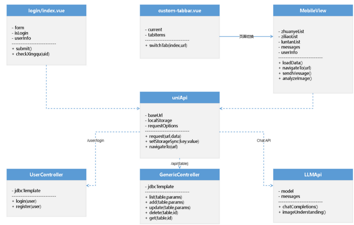
图 5-5 用户移动端模块类图
